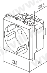
Méretetek / Dimensions (mm)
