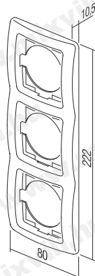
OE31 Függőleges / Vertical
