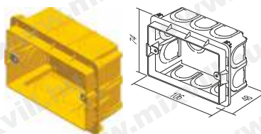
Típusok / types DM30 3M
