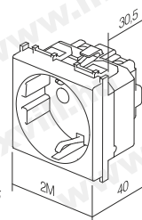
Méretetek / Dimensions (mm)
