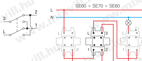
SE70 107 keresztkapcsoló / switch intermediate
