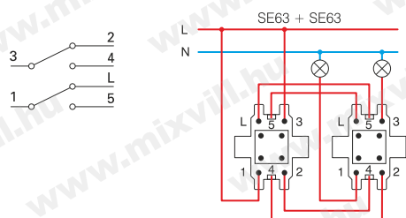
SE63 106 + 6 dupla váltókapcsoló / switch double 2 way
