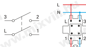
SE20 102 2 pólusúkapcsoló / 2 pole switch
