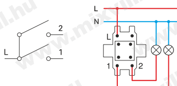
SE50 105 Csillárkapcsoló / switch 2 gang - 1way
