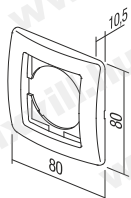
OE30 Vízszintes / horizontal
