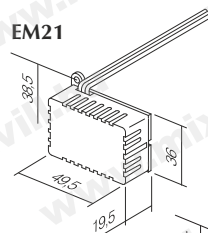
Méreték / Dimensions (mm)
