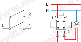
SE63 106 + 6 dupla váltókapcsoló / switch double 2 way
