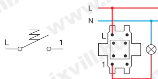
SE11 1 pólusú nyomógomb / 1 pole push button
