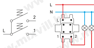
SE51 105 2 állású 1 pólusú nyomó / button 2 gang - 1way
