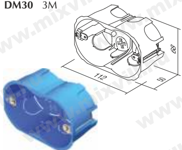
Típusok / types DM30 3M
